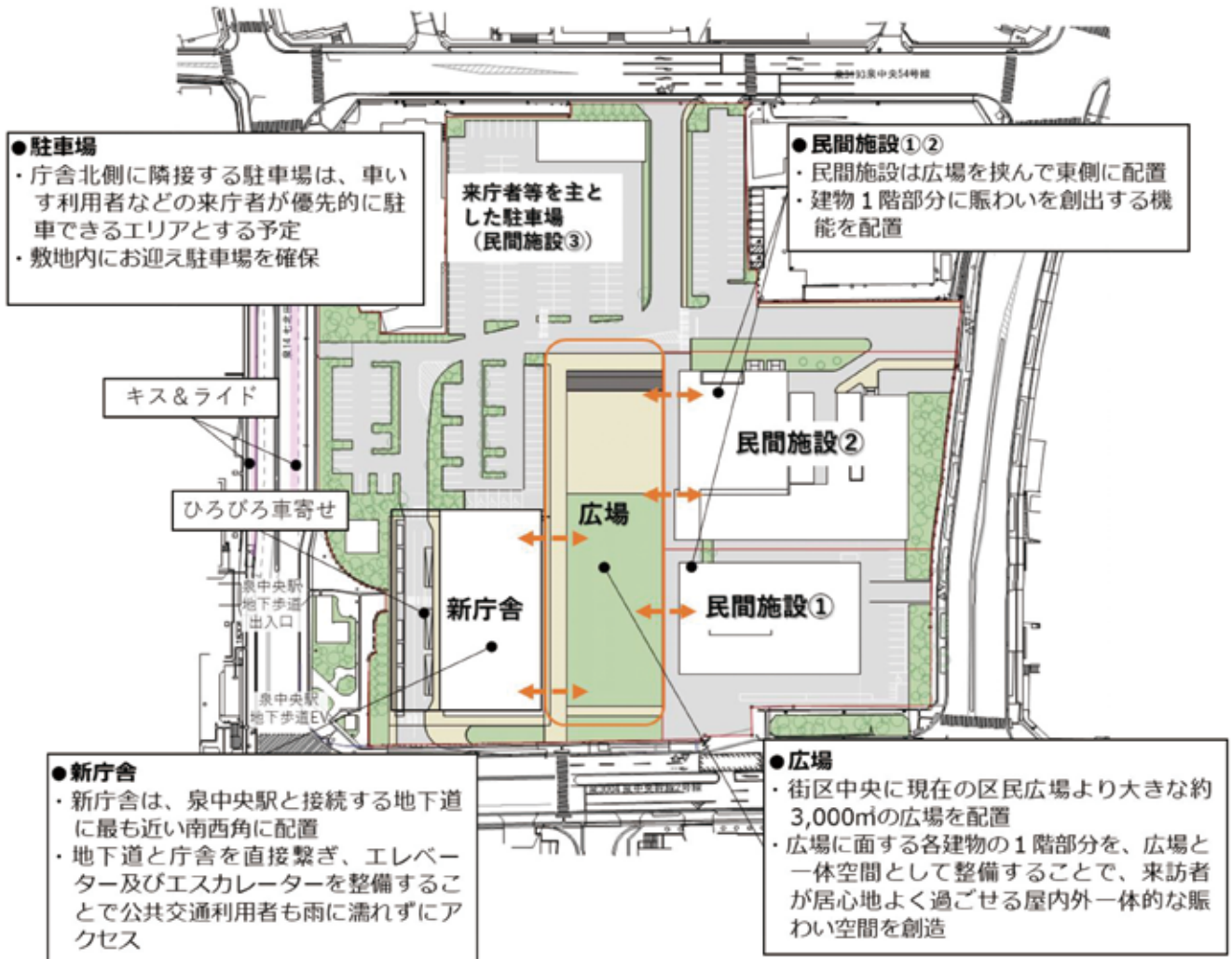
<図 配置図>
